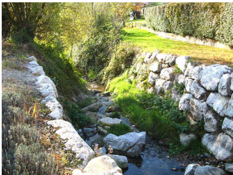
Hauteville-OT2 : Ruisseau de Lagnat, au Vernay – Enrochements de berges au niveau du pont situé vers le château.
