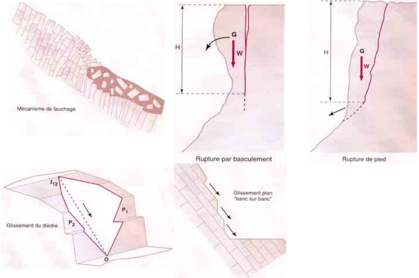
Figure 5 : Schémas présentant les principaux mécanismes à l'origine de chutes de blocs ou d'éboulements
